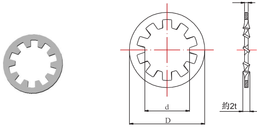
內齒形(A)
