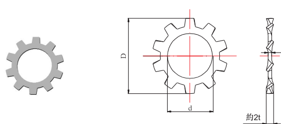
外齒形(B)
